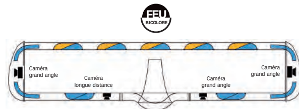
Modèle présenté : rampe VEGA avec sirène intégrée, défilement arrière (5 feux bicolores bleu/orange) et vidéo (4 caméras intégrées).
