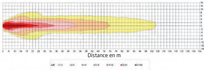
DIAGRAMME HORIZONTAL D'ÉCLAIRAGE
