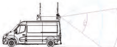
Angle de vision vertical des caméras : Caméra vision proche 120° / Caméra vision lointaine 45°
